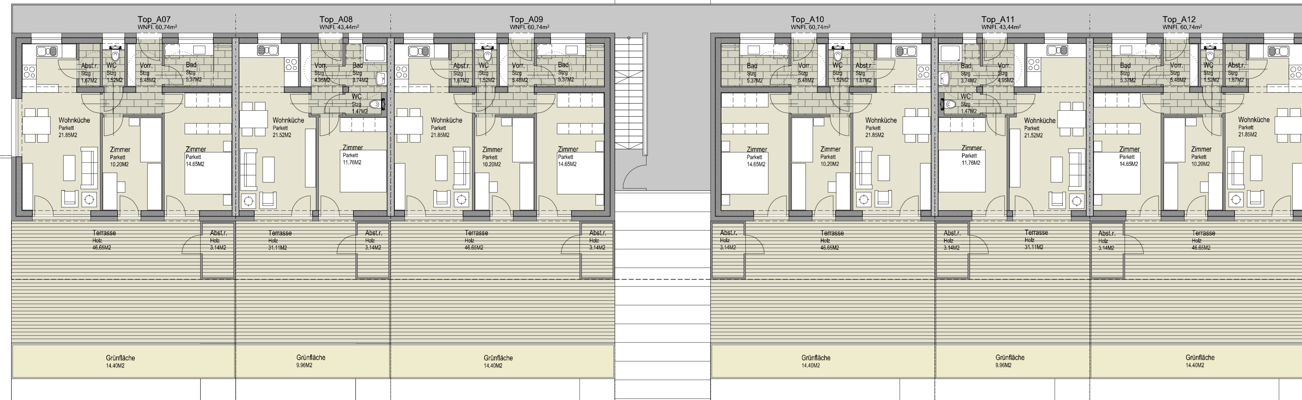
HAUS A WNFL 1.OG : 329,84m 2
